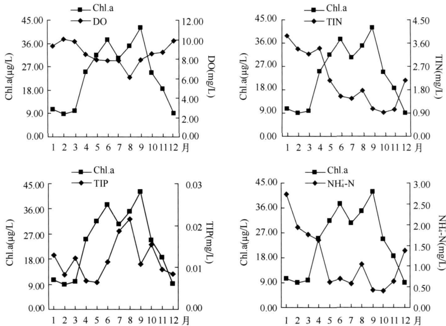
图 6 梅梁湾、贡湖、竺山湾 Chl a 与水质指标的关系
