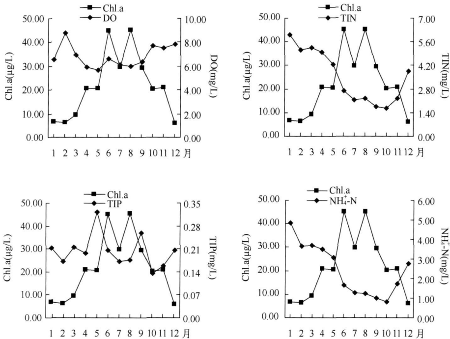
图 7 入湖口 Chl a 与水质指标的关系
