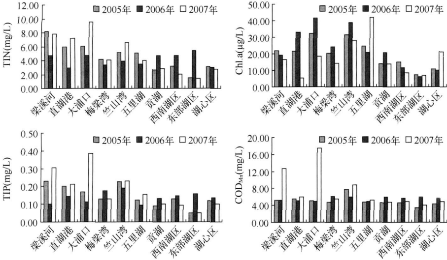
图 3 不同湖区水质指标年平均值 (2005-2007年)
