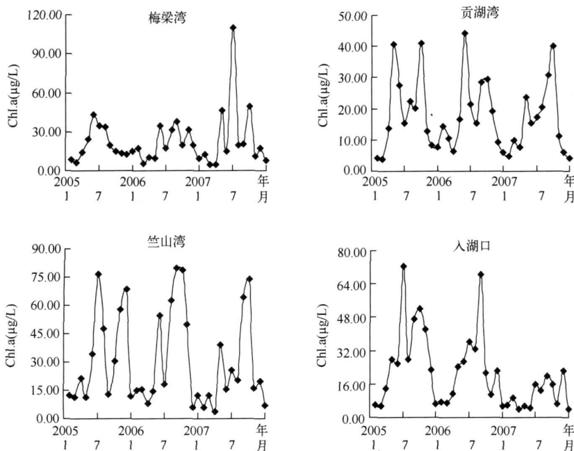
图 5 2005-2007年典型湖区 Chl a的时间变化
