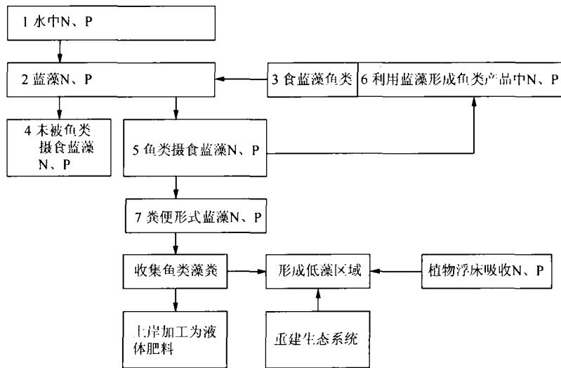
图6 鱼类控制蓝藻存在的问题及解决途径
