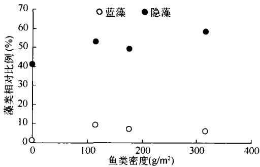
图 3 鲢鱼密度对蓝藻和隐藻相对比例的影响 (根据唐汇娟 2006 年在武昌东湖实验数据)
