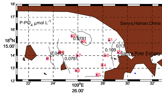
(d) Spatial distribution of the annual concentration of \text{P-PO}_4 .
